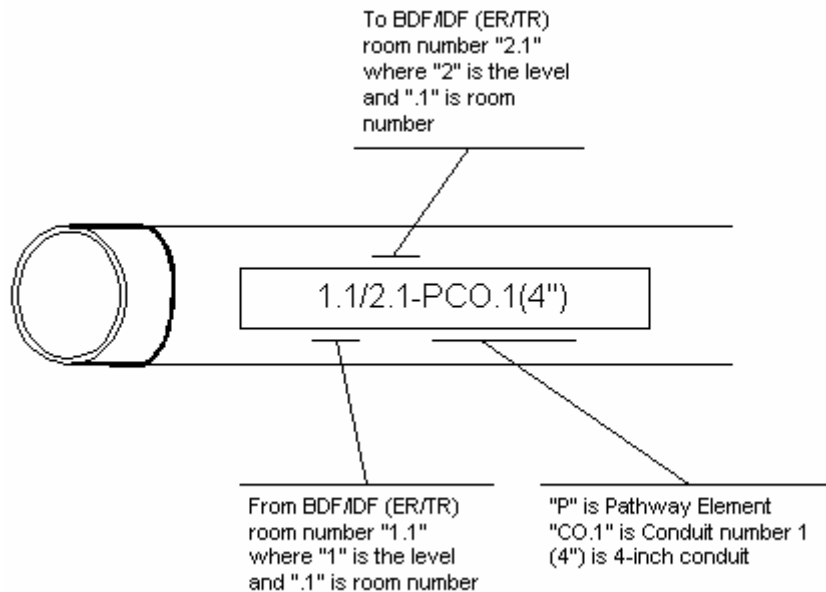
Figure 4-3 Conduit Labeling
